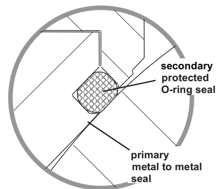
PMSS 雙重密封示意
