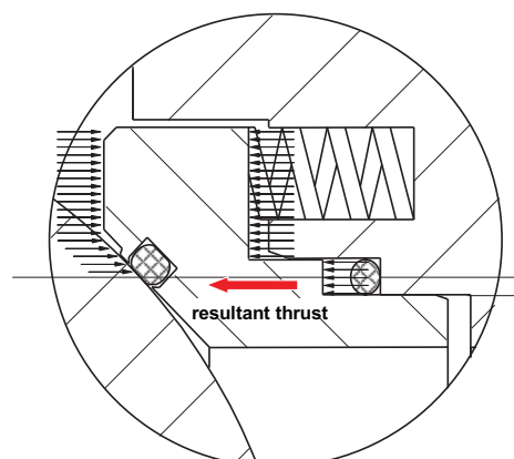
下游閥座
