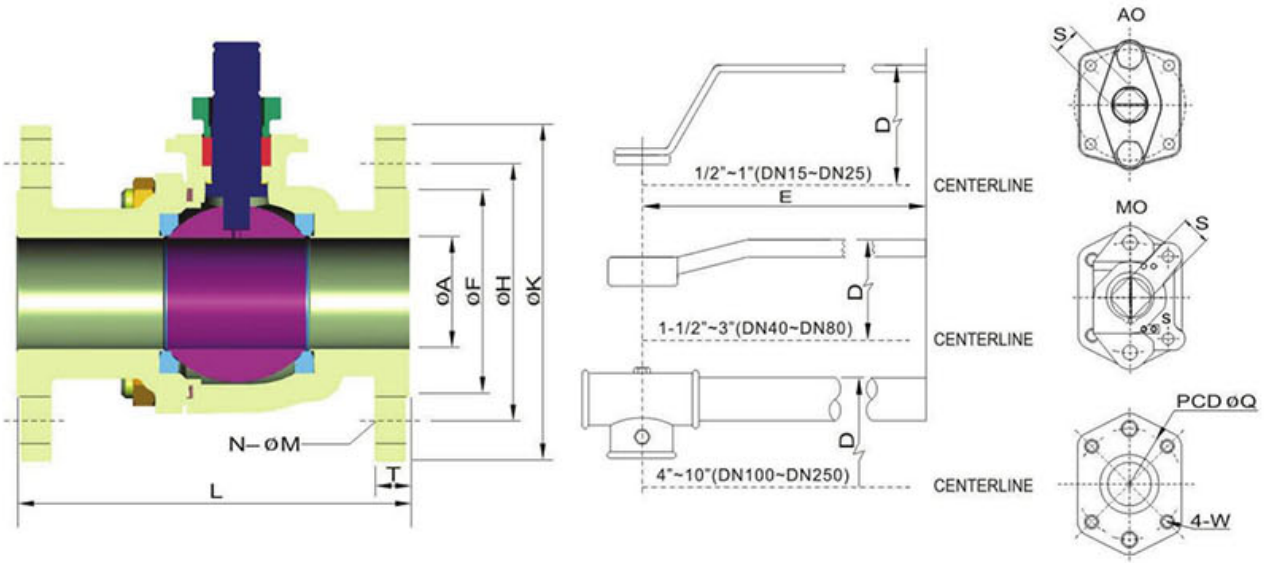
DIMENSIONS (JBF-A1 SERIES JIS 10K)
