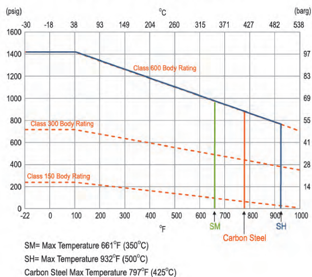
JBT-M 2"~24" (DN50~DN600)
