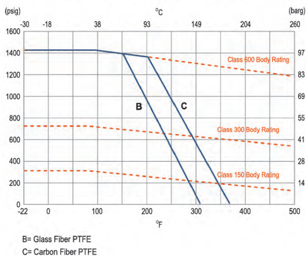
JBT-F 2"~24" (DN50~DN600)
