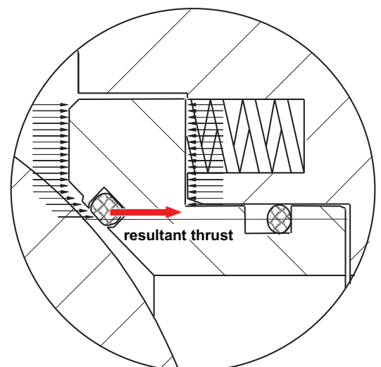
下游閥座
