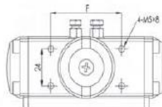
JEW-032
