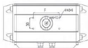
JEW/JEV-050-190
