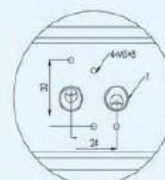
JEW/JEV-050-210
